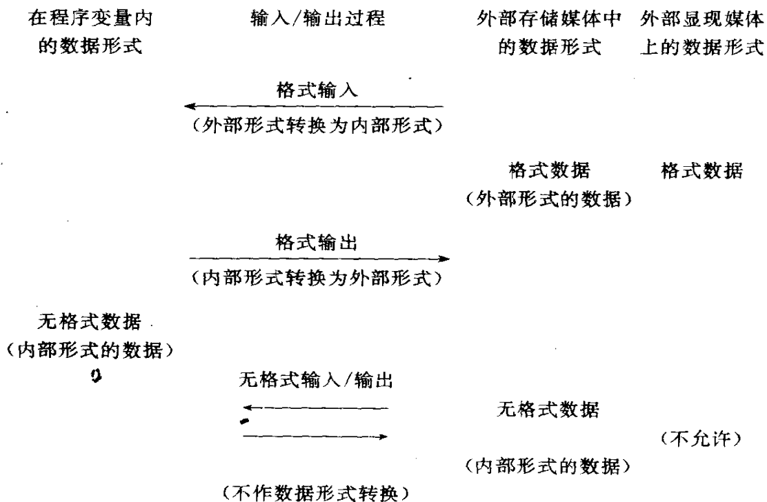
图 8.1 输入/输出过程中的数据形式转换
